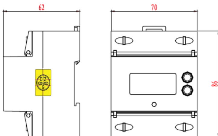
Fig. 2: Abmessungen Gehäuse
