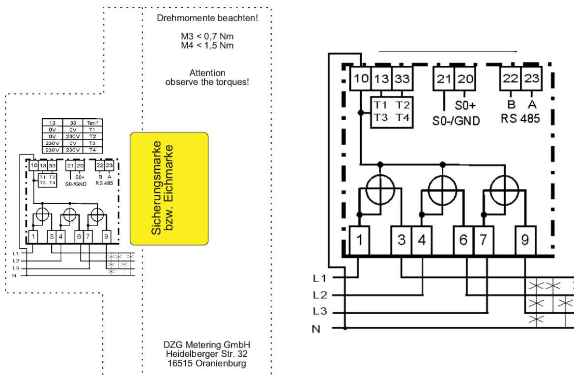
Fig. 4: Schaltbild
