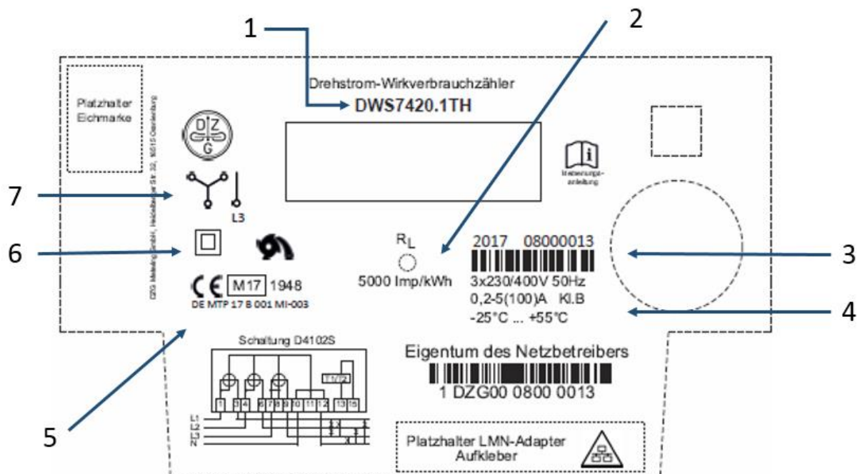
Abbildung 9 Leistungsschild
