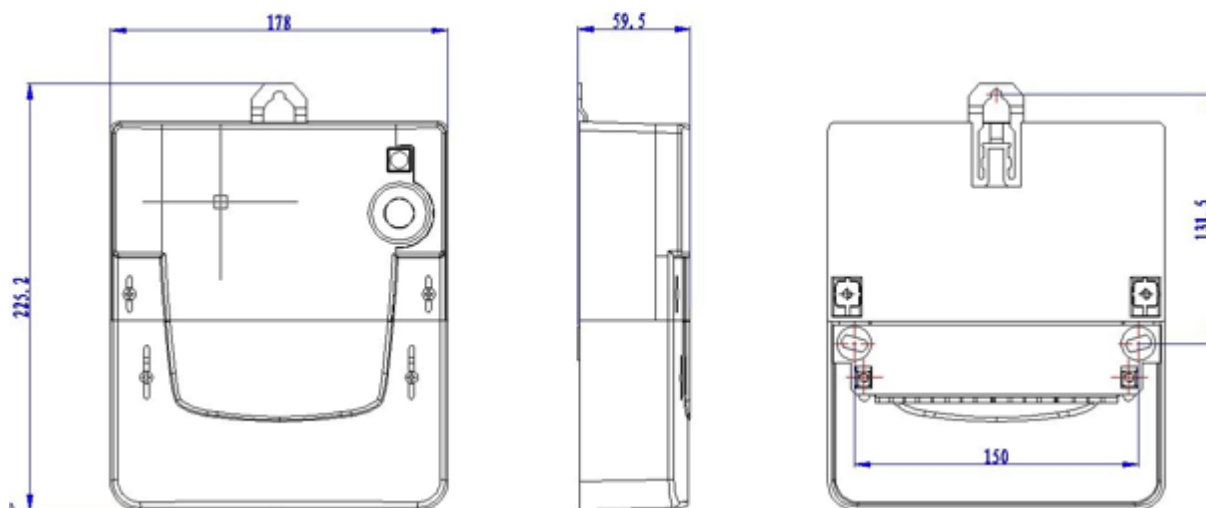
Abbildung 2 Abmessungen Gehäuse
