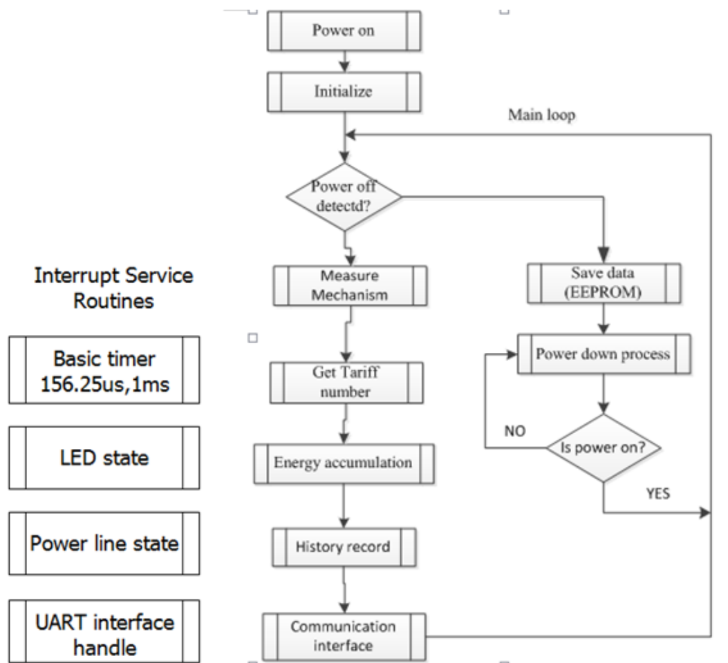
Abbildung 14 Firmware Flussbild
