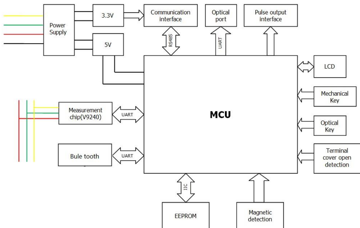
Abbildung 12 Blockdiagramm DVS74.G2
