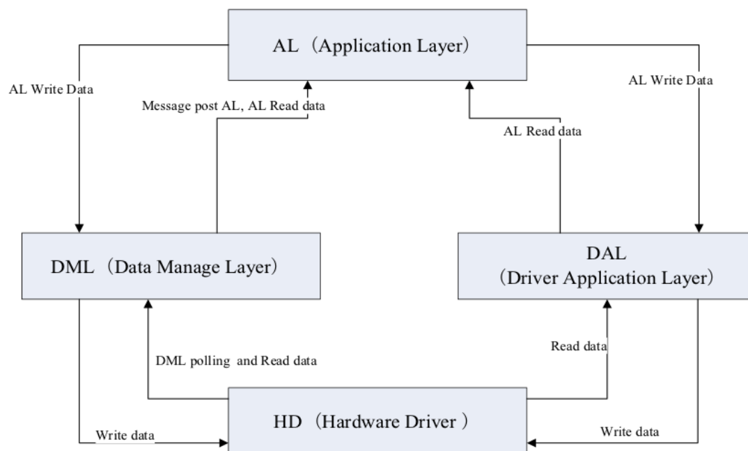
Abbildung 13 Struktur der Firmware
