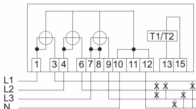
Abbildung 5 Schaltbild
