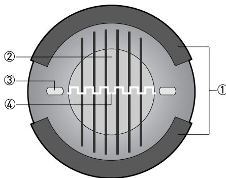
Figuur 6-1: Meetprincipe
