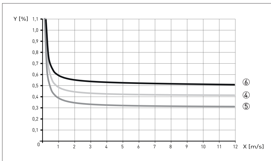
Figuur 6-5: Stroomingssnelheid t.o.v. nauwkeurigheid X [m/s]: flowsnelheid Y [%]: afwijking van de werkelijk gemeten waarde (mw)
