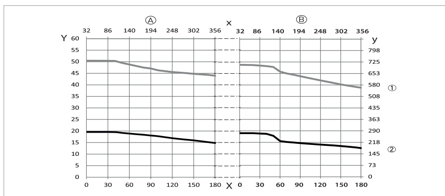
Figuur 6-7: Drukvermindering; ANSI B16.5
