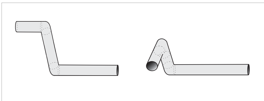
Figuur 3-5: Inlaat wanneer er 2- en/of 3-dimensionele bochten worden gebruikt voor de flowmeter
